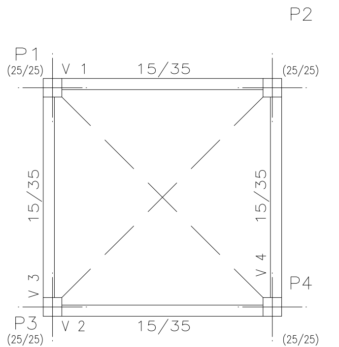
Planta de Forma vigas de travamento escala → 1/50
