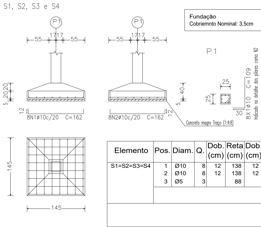
Detalhamento de Sapatas escala → 1/50
