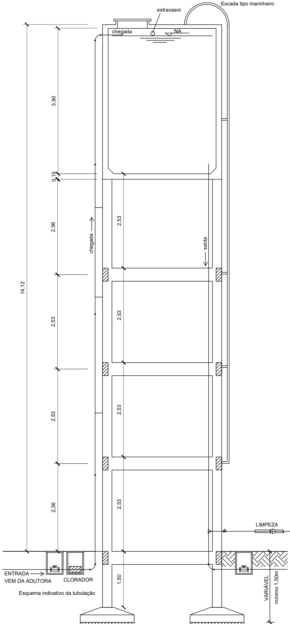
Seção da estrutura escala → 1/50
