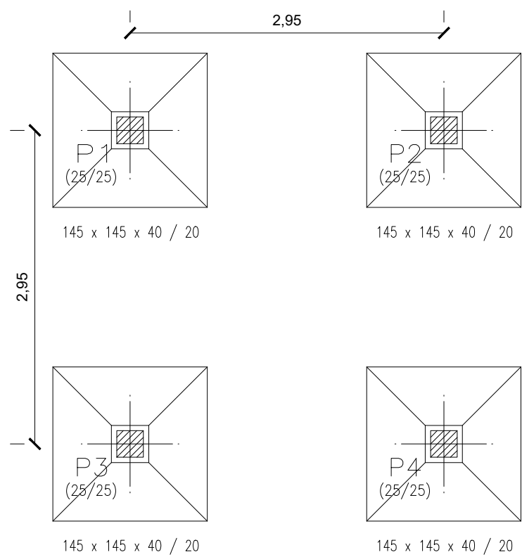
Planta de Forma das fundações escala → 1/50
